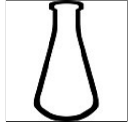
Erlenmeyer Flask
